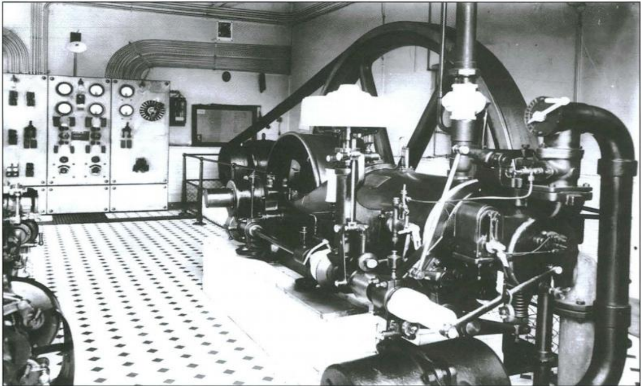
Twee grote dieselmotoren, met elk één cilinder, uit de Bollinckxfabriek uit Huizingen, voorzagen het sanatorium van stroom. De dynamo's achteraan in de kamer werden aangedreven met een drijfriem. Omstreeks 1950. (Verzameling Dr. Paul Dierckx)
